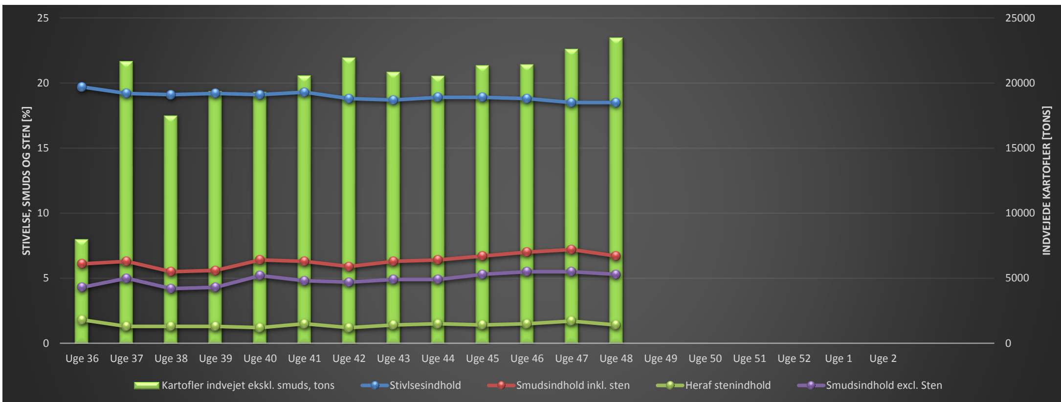
Figuren viser udviklingen i kampagnen 2017. De grønne søjler viser den indvejede mængde kartofler per uge (excl. smuds). Den blå graf viser stivelsesprocenten i de indvejede kartofler i den pågældende uge. Den røde graf viser smudsprocenten inkl. sten, den lilla graf viser smudsprocenten excl. Sten, mens den grønne graf viser stenprocenten.
